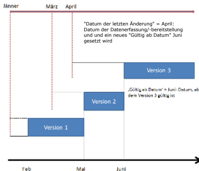
Abbildung 8: Versionierung - Version 3
